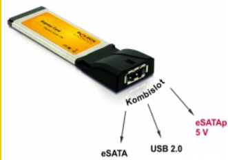
eSATAp (Power Over eSATA)
